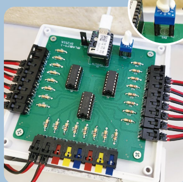
Wi-Fi内蔵本体 自動販売機の内部庫内へ設置
