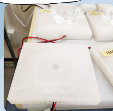
センサートレイ 専用ケーブルを配線してロッカー内へ設置
